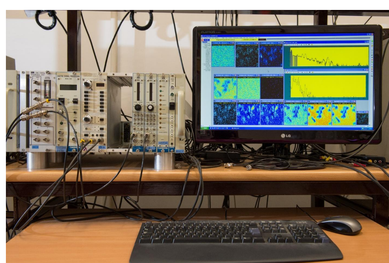
A pásztázó ionmikroszkop mérésvezérlő-adatgyjtő rendszere (2013)
